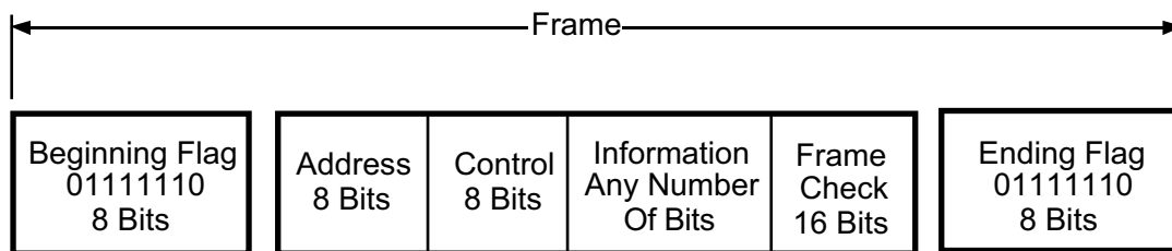
SDLC Message Format
