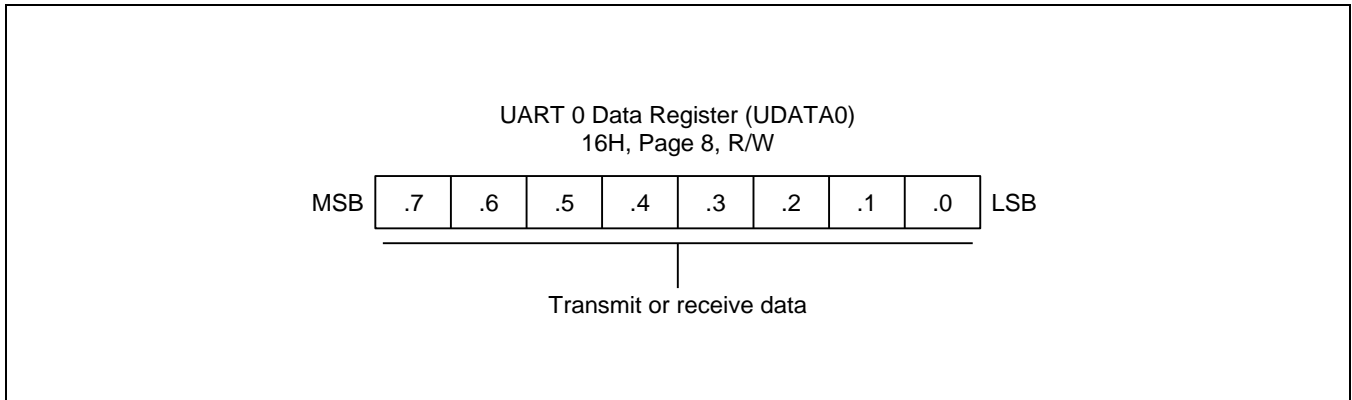
Figure 20-3 UART 0 Data Register (UDATA0)
