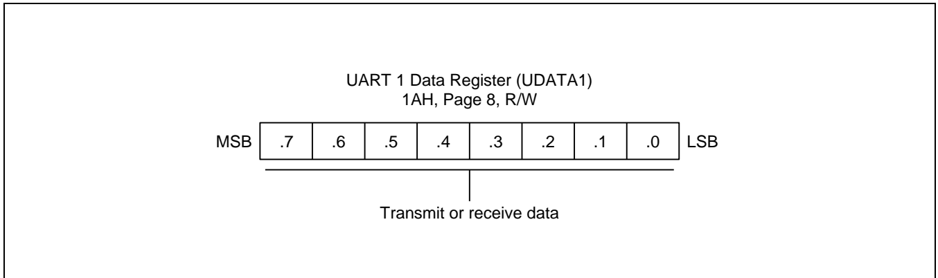
Figure 21-3 UART 1 Data Register (UDATA1)
